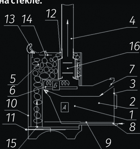
Рисунок 1. Конструкция банной печи серии ПС
