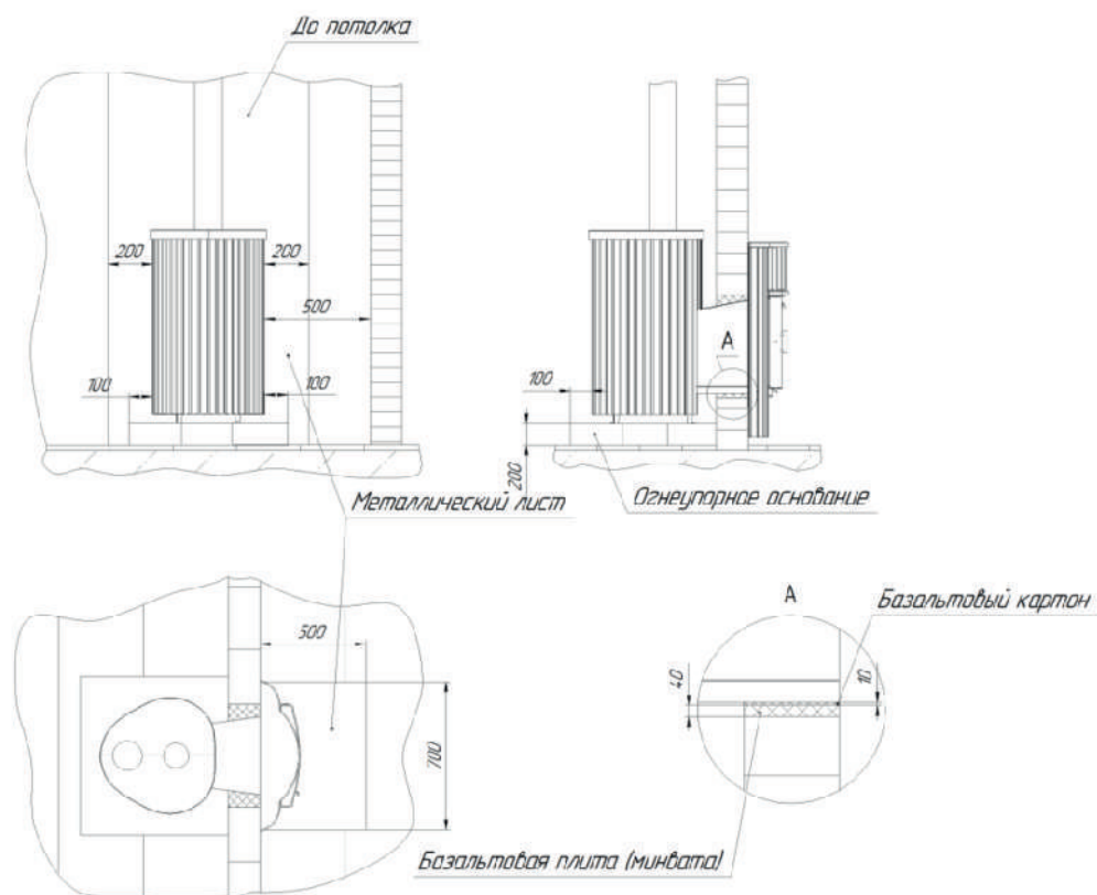
Рис.№ 3 Схема установки банной печи «Мини», «Малютка», «Оптим», «Квадра», «Макс» (серии ПФ) на минимально безопасном расстоянии от несущих и ограждающих конструкций.
